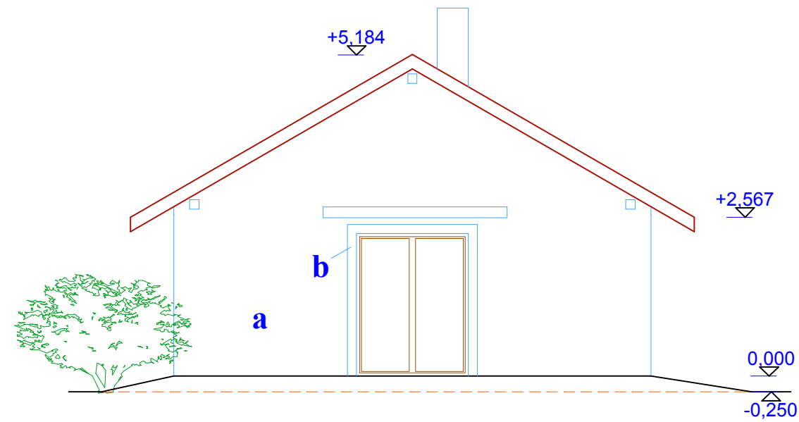
POHLED BOČNÍ
