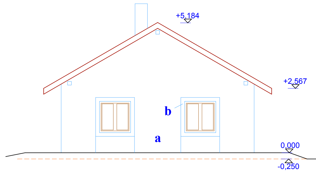
POHLED BOČNÍ
